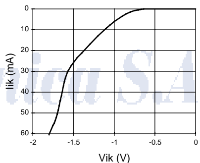
Input Clamp (Vik)
